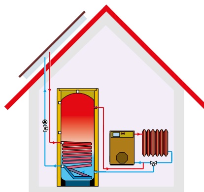
Einbindung über Rücklaufanhebung
