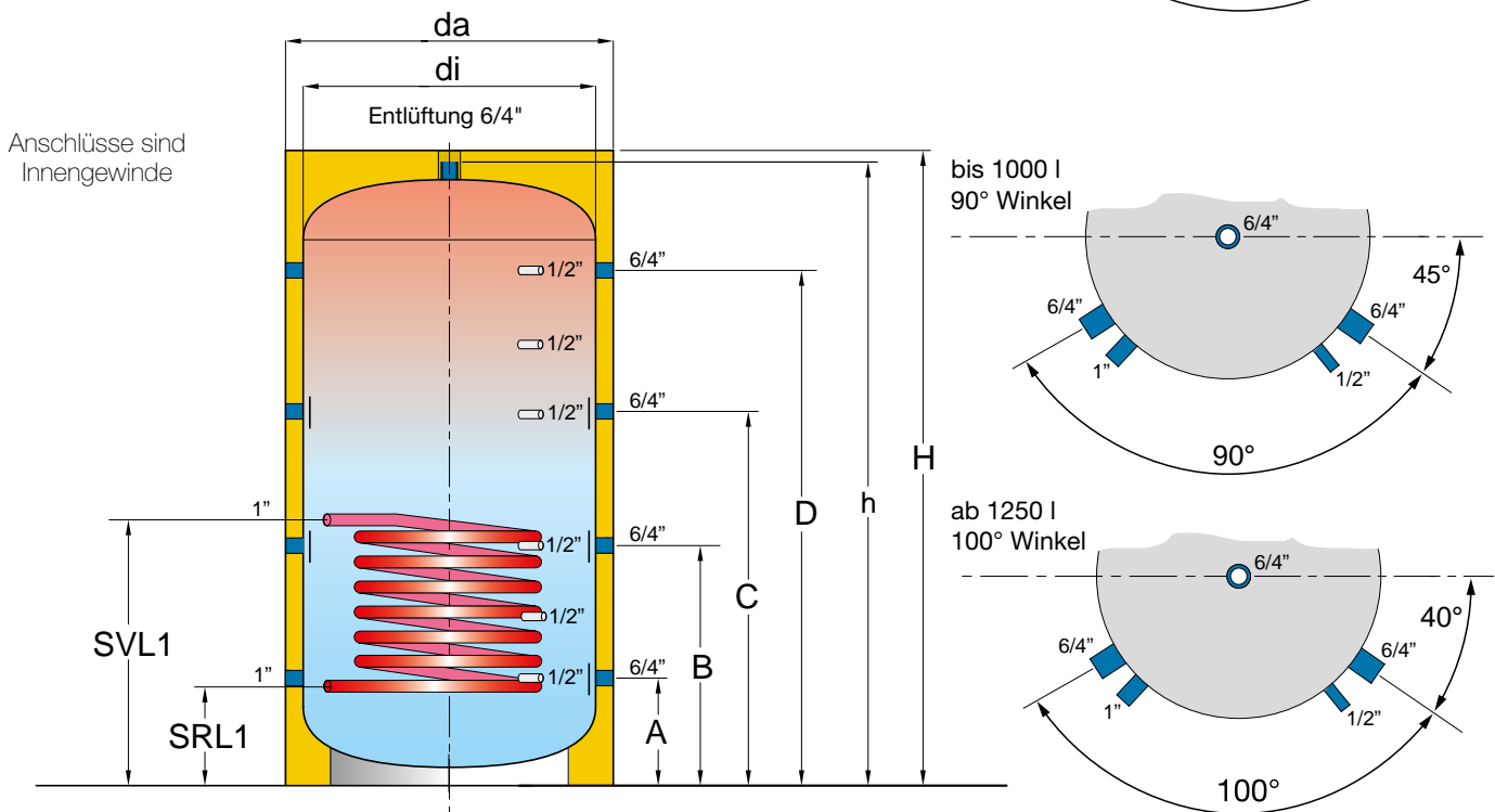
Pufferspeicher ohne bzw. mit einem Solarregister
