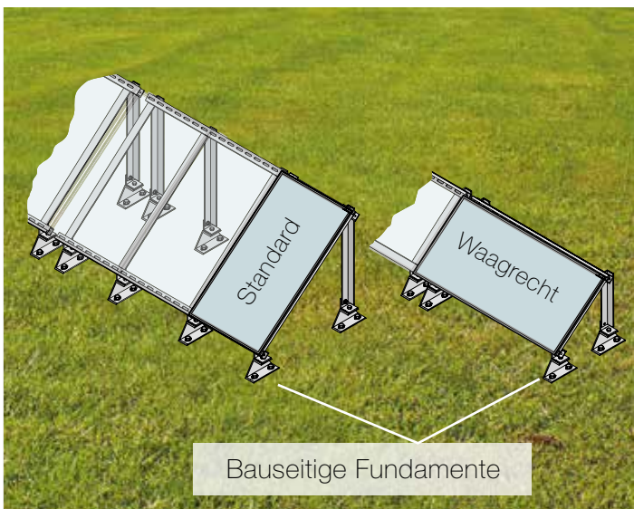
Freiaufstellung für CPC und Sunny line 45° und 70°
